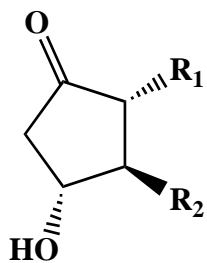
PGE
