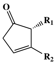
PGC
