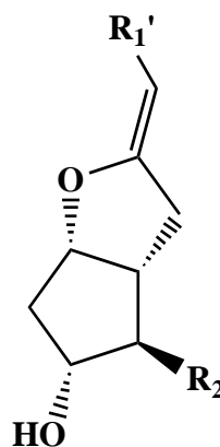
PGI
