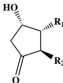
PGD
