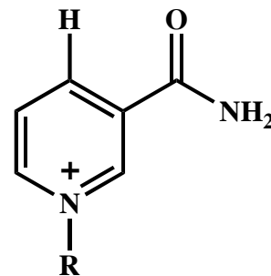
NADP +
