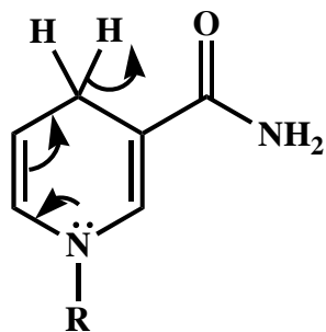
NADPH
