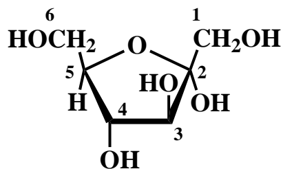
\alpha -D-fructofuranose
