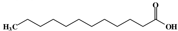
lauric acid (12:0)
