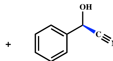
( R )-mandelonitrile
