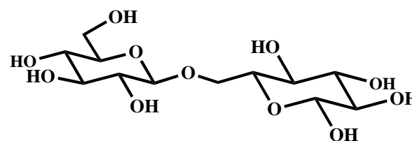
gentiobiose
