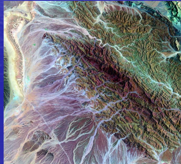
Geology of Oman (Landsat)
