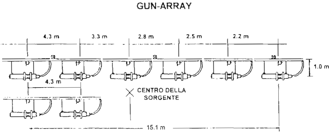
CONFIGURAZIONE DI MULTIPLE SORGENTI "AIR-GUN"
