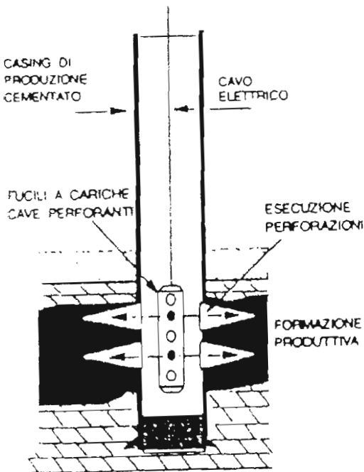
PERFORAZIONE CASING DI PRODUZIONE
