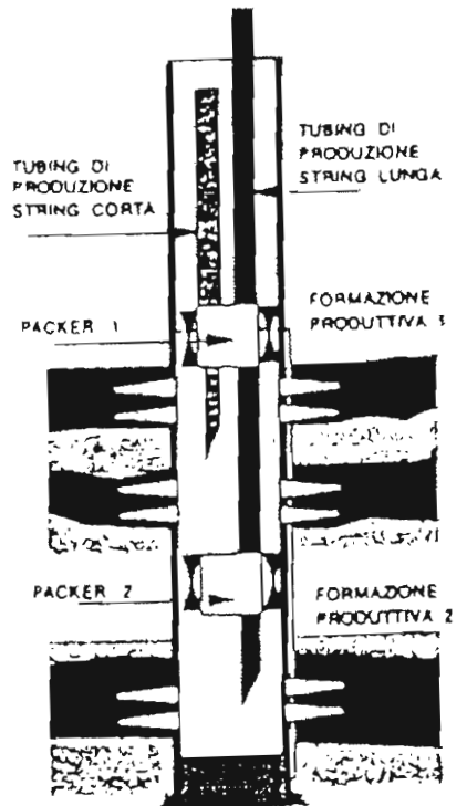
COMPLETAMENTO DOPPIO CON CASING TUBATO E PERFORATO
