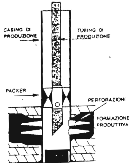
COMPLETAMENTO CON CASING TUBATO E PERFORATO
