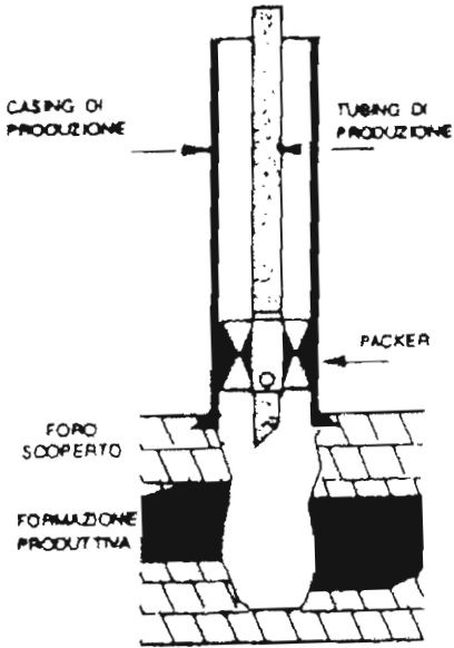
COMPLETAMENTO IN FORO SCOPERTO
