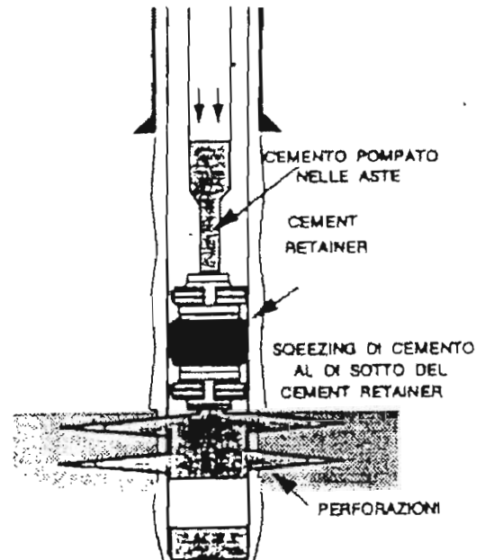
CEMENTAZIONE INTERVALLI TESTATI IN FORO TUBATO
